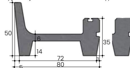
Type 50.4 jeune bétail
