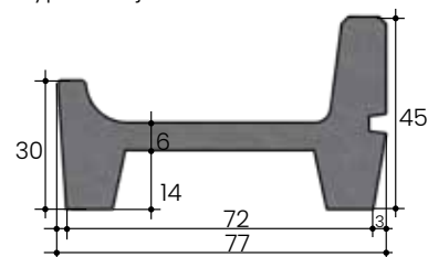
Type 30.4 jeune bétail
