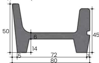
Type 30 jeune bétail Type 30.3
