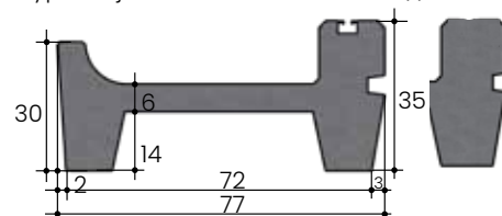
Type 30.4 jeune bétail
