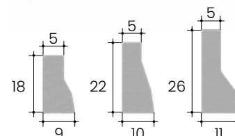
Dimensions du trou
