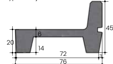
Type 20.4 jeune bétail
