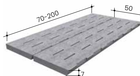
Type 17/05 avec 5% surf. d'écoulement
