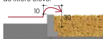
Elément en L
