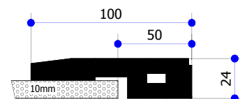
42.420354 Gummiabschlussprofil zu ebener Fläche
