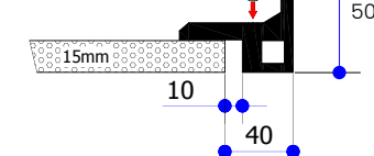
45.420350 Profilé d'angle en caoutchouc pour raccord mural
