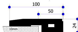
42.420354 Profil d'assemblage en caoutchouc pour raccorder la surface plane
