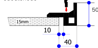
45.420350 Raccord de paroi en caoutchouc
