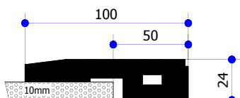
Profil d'assemblage en caoutchouc pour raccorder la surface plane
