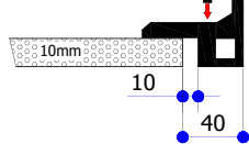
Profilé d'angle en caoutchouc
