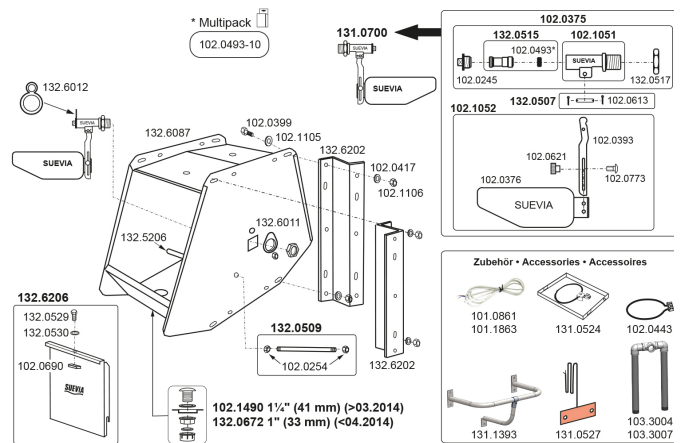
130.0620 Mod. 620 (> 11.2010)
