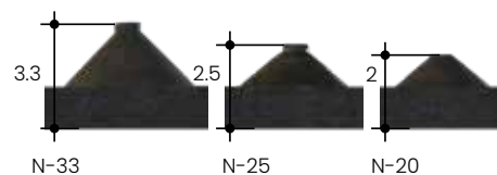
HAUTEUR N-33/N-25/N-20
