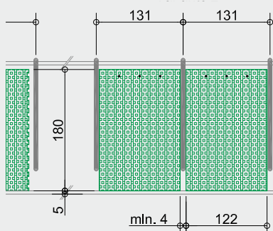
MONTAGEBEISPIEL EINZELMATTE
