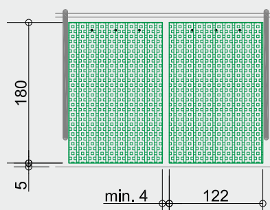
MONTAGEBEISPIEL
