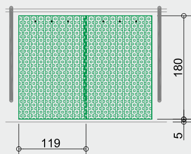
MONTAGEBEISPIEL PUZZLEMATTE
