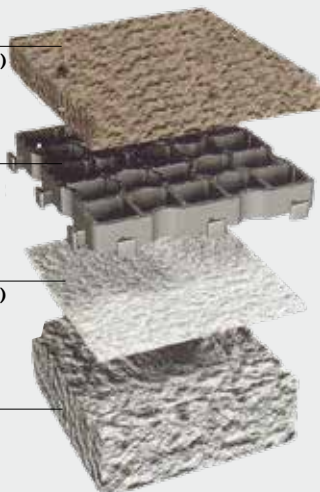
Befüllung (Sand/Humus)
