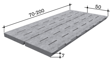
Typ 17/05 mit 5% Durchlass
