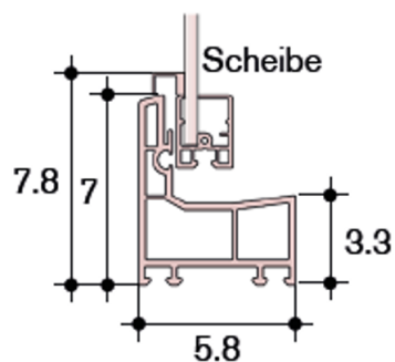
Querschnitt Fenster
