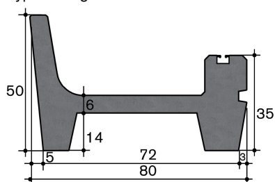
Typ 50 Jungvieh
