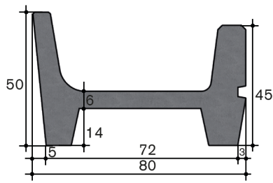
Typ 50.4 Jungvieh
