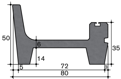
Typ 50 Jungvieh
