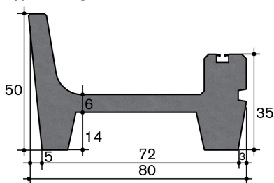
Typ 50 Jungvieh
